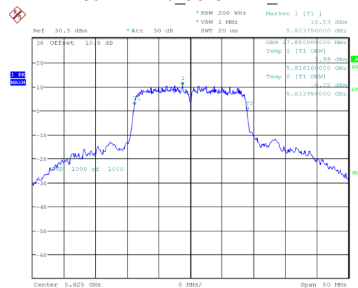
802.11ac20_5825MHz_Chain 1
