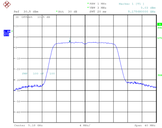
802.11ac20_5180MHz_Chain 0
