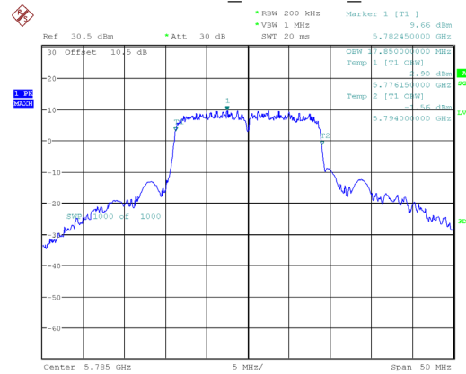
802.11ac20_5785MHz_Chain 0
