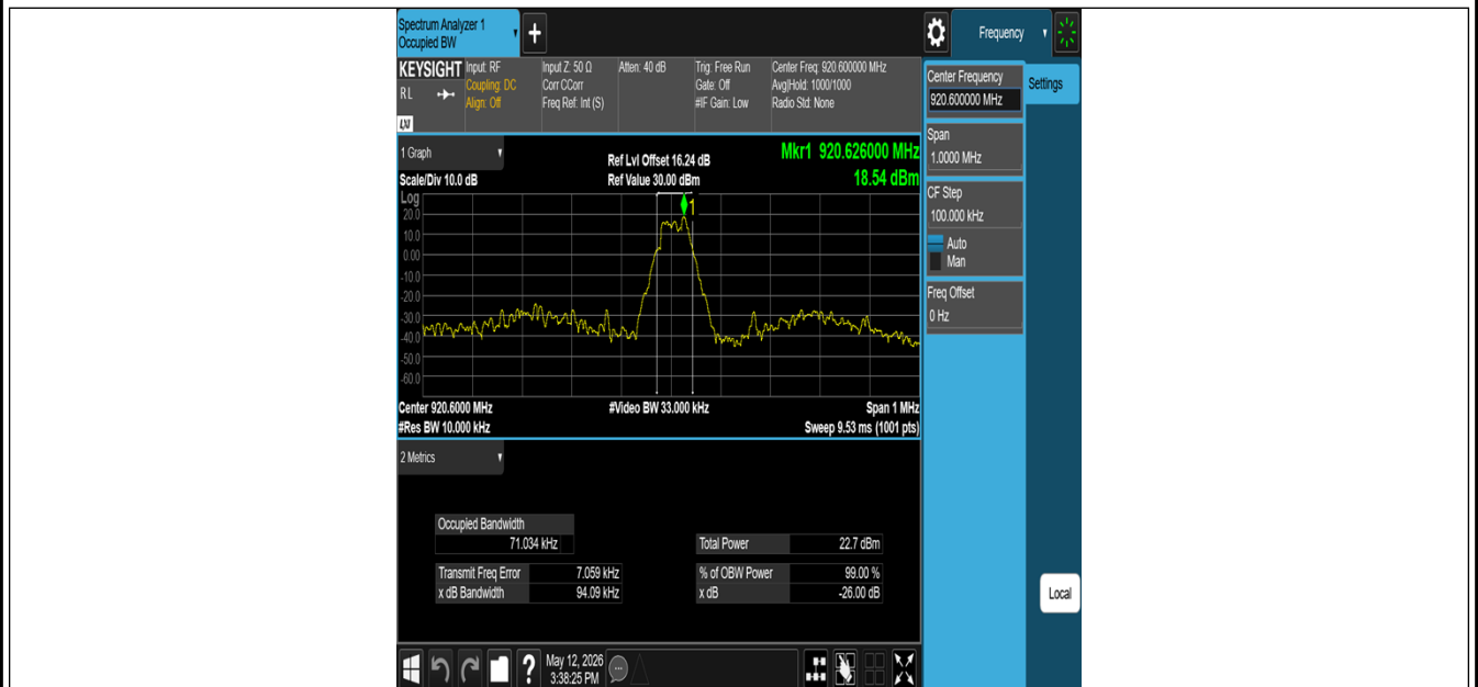
SUB-1G-Ant1-920.6
