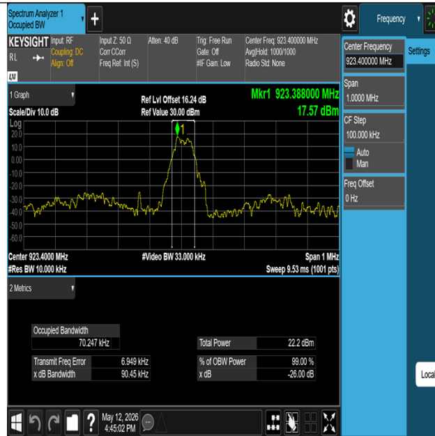
SUB-1G-Ant1-923.4
