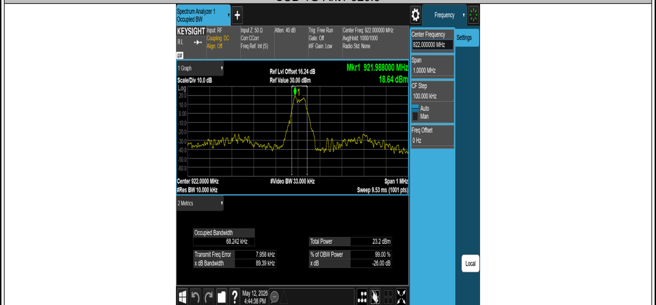
SUB-1G-Ant1-922
