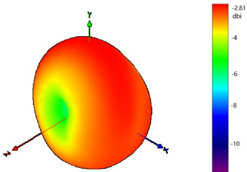
Horizontal 2400MHz
