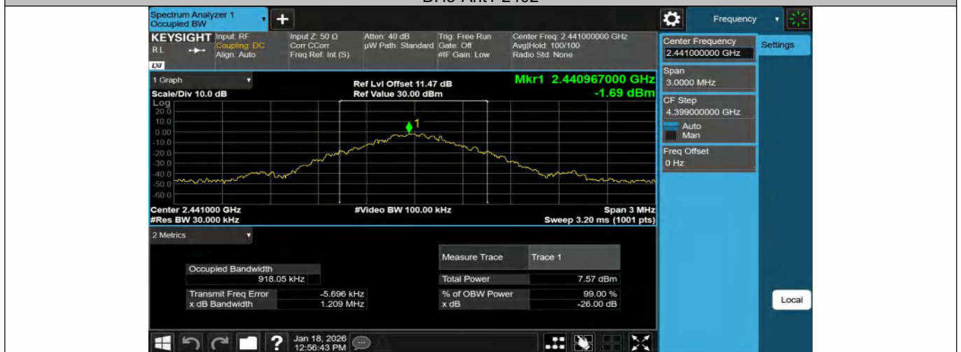
DH5-Ant1-2441
