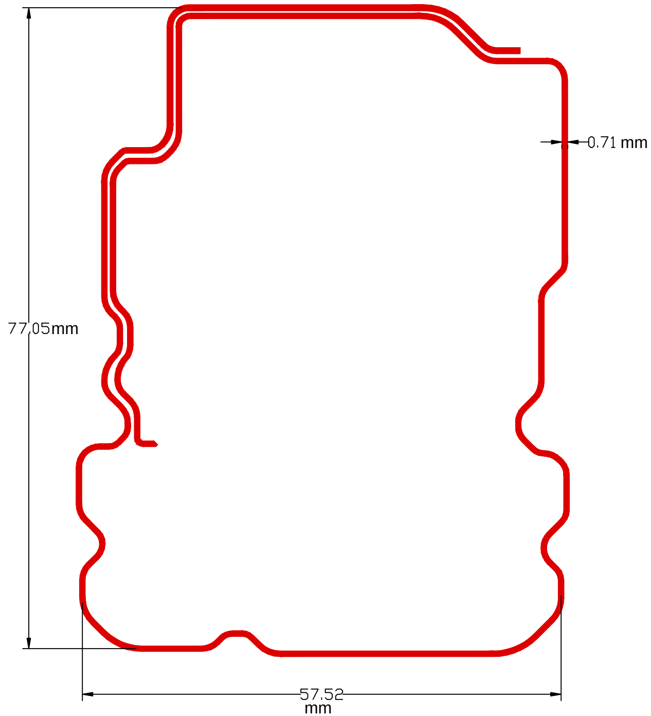
MP200 NFC Antenna
