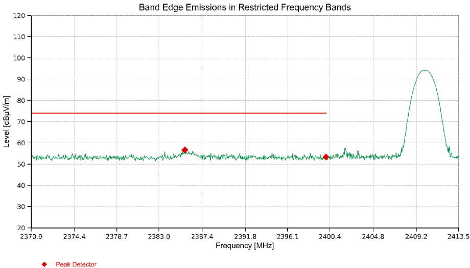
SRD_ANT1_2410_1Mbps
