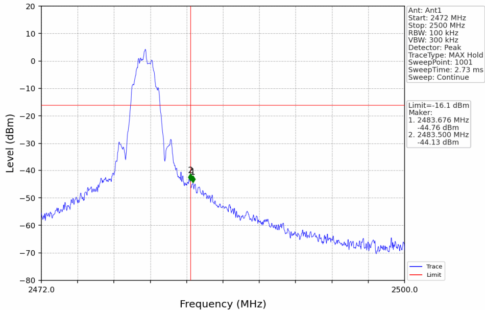
2M_HCH_2480MHz_Ant1_NTNV
