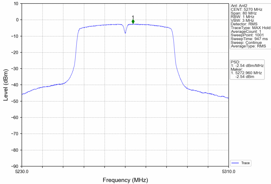
802.11n(HT40)_LCH_5270MHz_MIMO_NTNV
