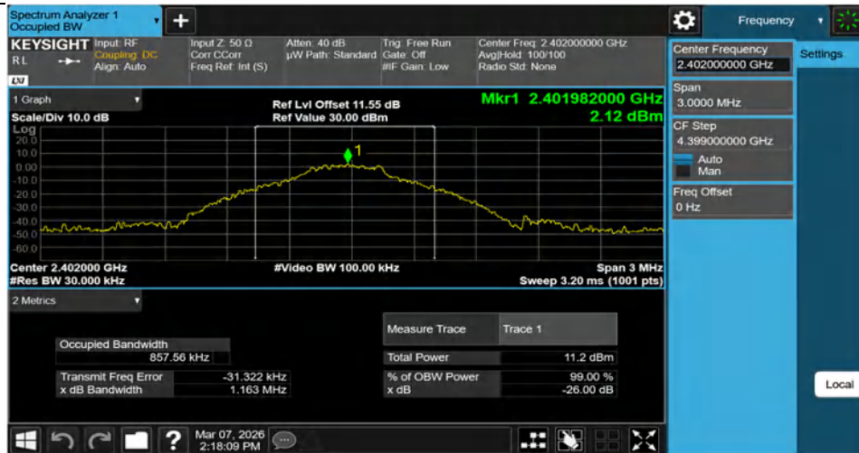
DH5-Ant1-2402
