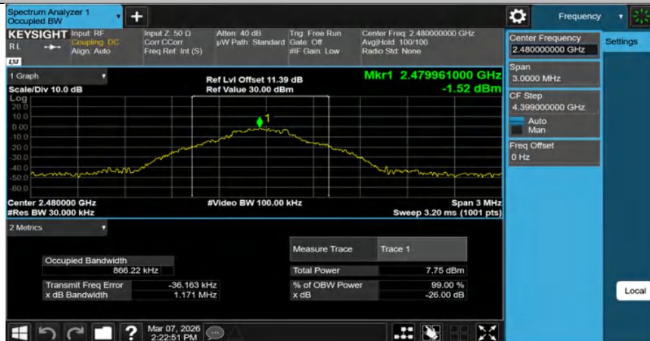
DH5-Ant1-2480
