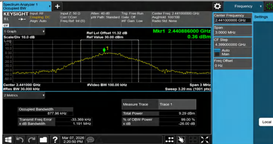
DH5-Ant1-2441
