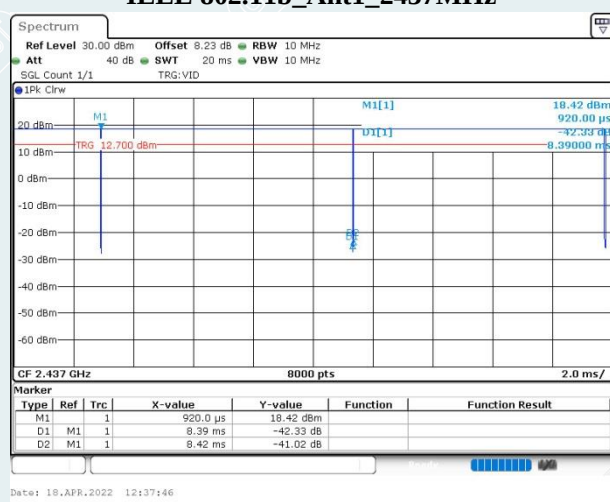
IEEE 802.11b_Ant1_2437MHz
