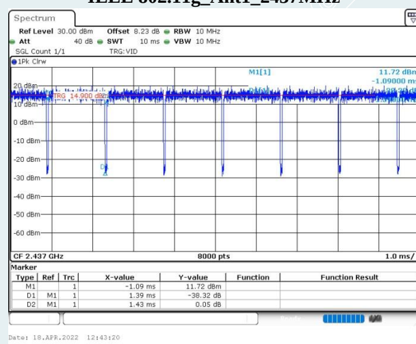
IEEE 802.11g_Ant1_2437MHz
