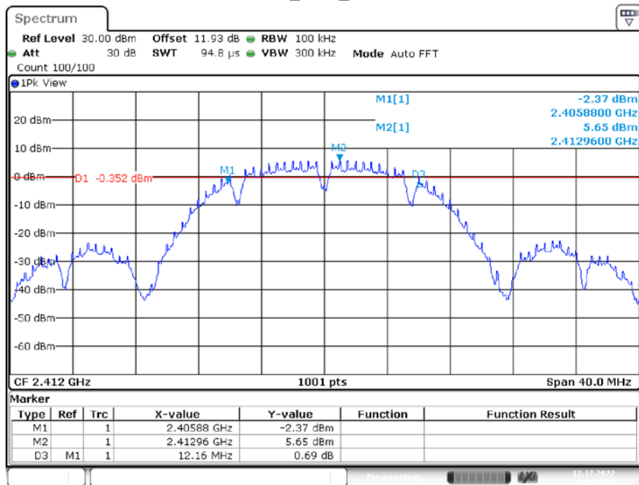
11B_Ant1_2412
