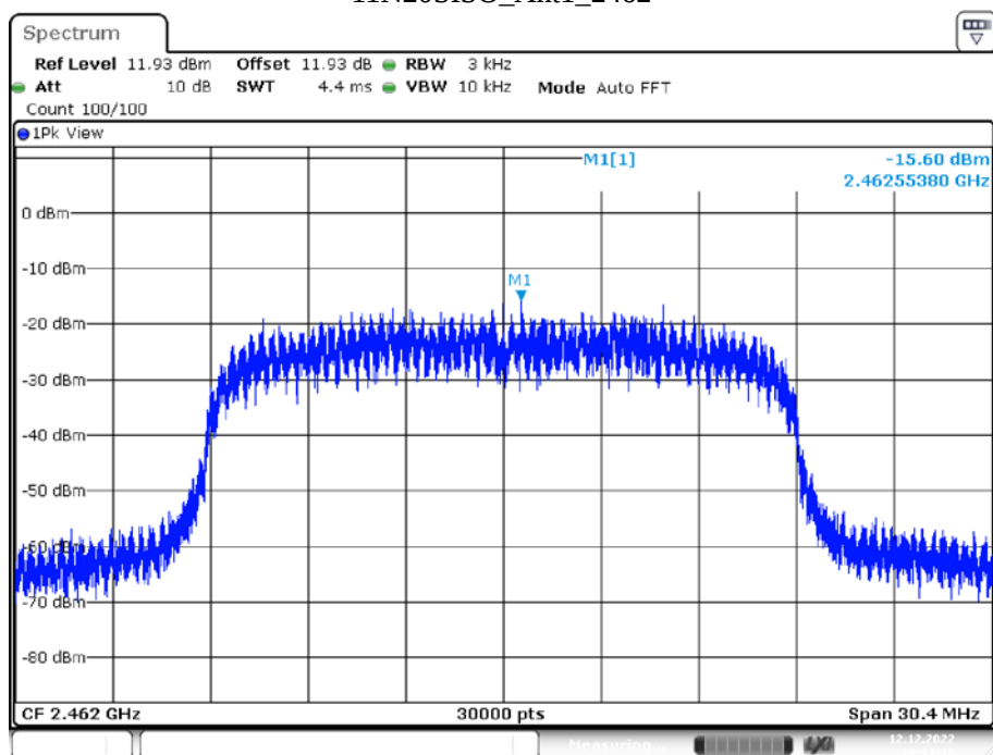
11N20SISO_Ant1_2462
