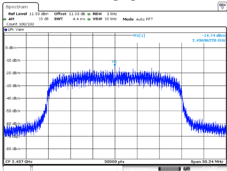
11N20SISO_Ant1_2437
