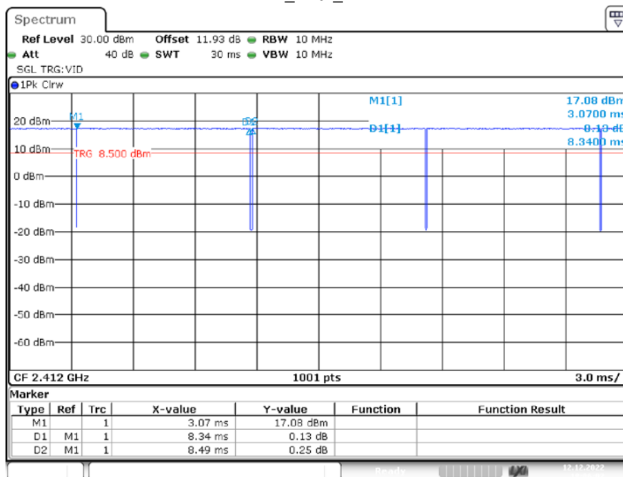
11B_Ant1_2412
