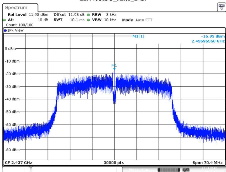
11N40SISO_Ant1_2437
