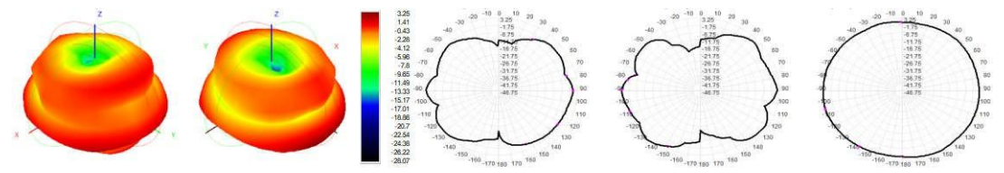
ANT-2-5G
