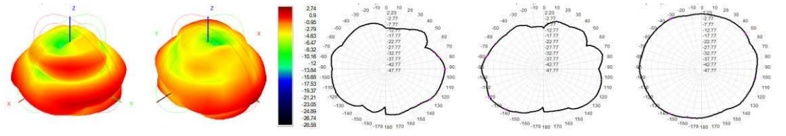
5850 3D-E1-E2-H
