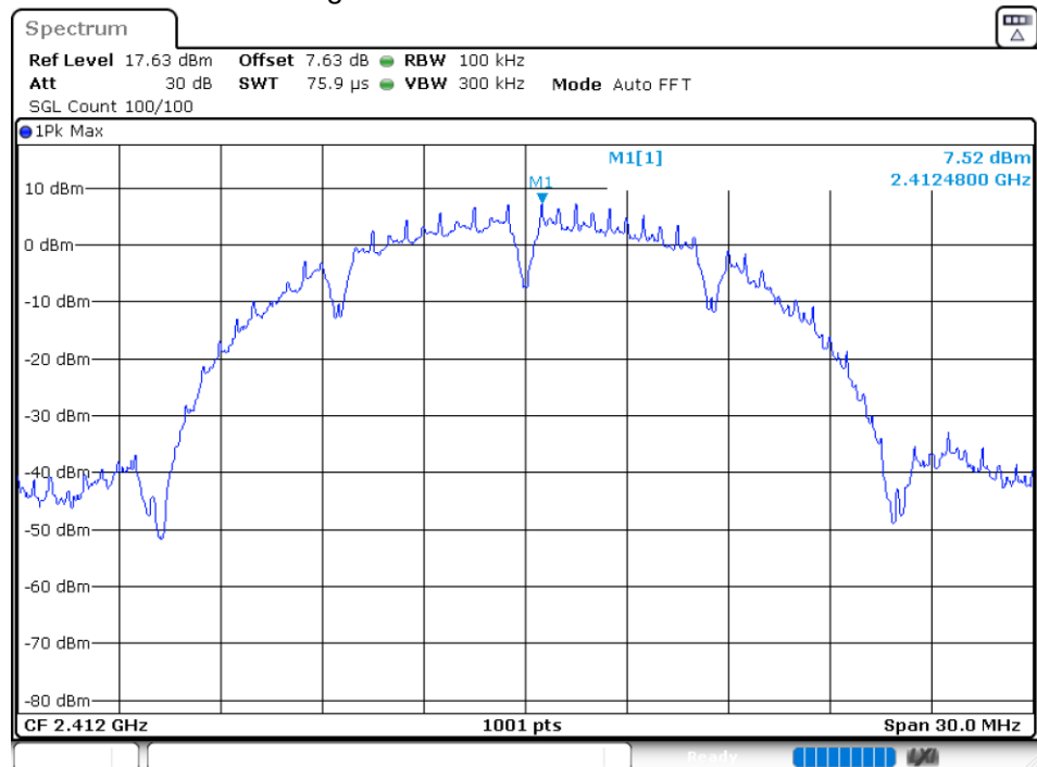
Band Edge NVNT 802.11b 2412MHz Ant 1 Ref
