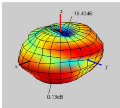
2436.000MHz
