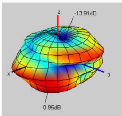
2400.000MHz
