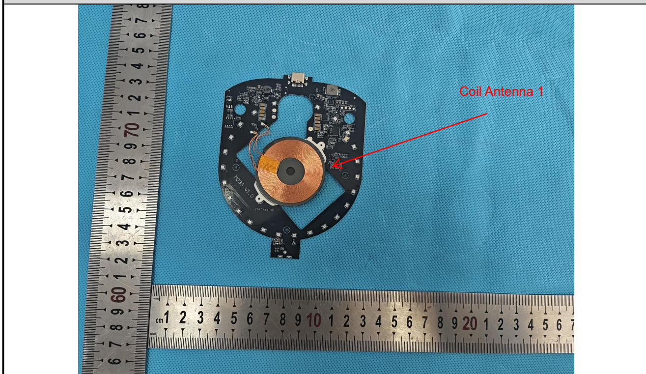
EUT Photo
