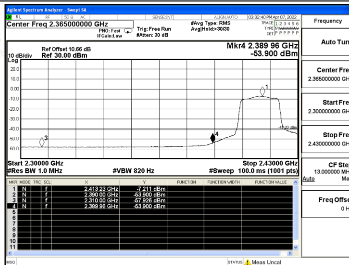
11AX20SISO_Ant B_Low_2412_AV
