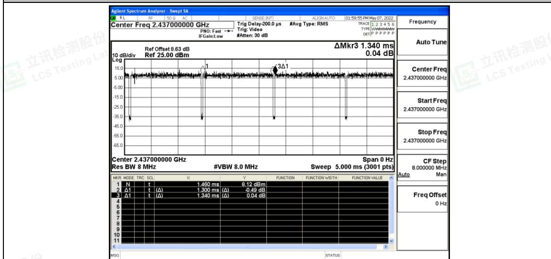
11AX20SISO_Ant B_2437
