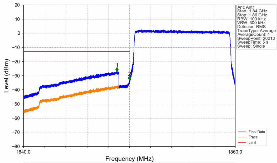
Band2_10MHz_QPSK_LCH_1855MHz_RB_50_0_NTNV
