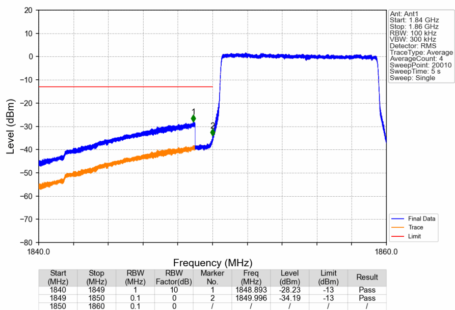
Band2_10MHz_16QAM_LCH_1855MHz_RB_50_0_NTNV
