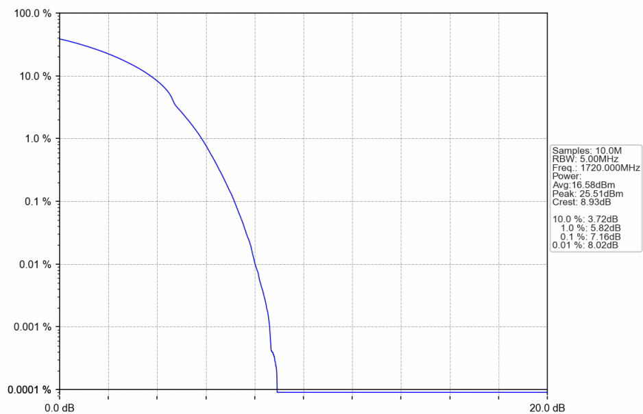
Band66_20MHz_16QAM_LCH_1720MHz_RB_100_0 NTN
