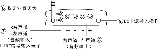
后视图
