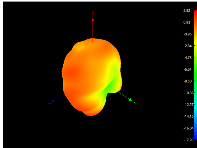
2400MHz
