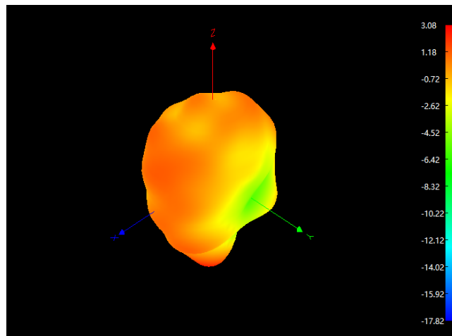
2450MHz
