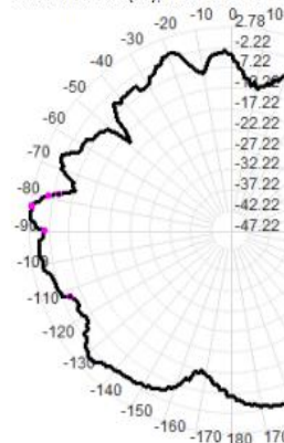
5850.0MHz Total(E1), Max= 2.52dBi
