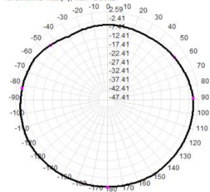
5150.0MHz Total(H), Max= 2.36dBi
