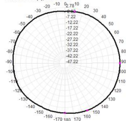
5850.0MHz Total(H), Max= 2.78dBi
