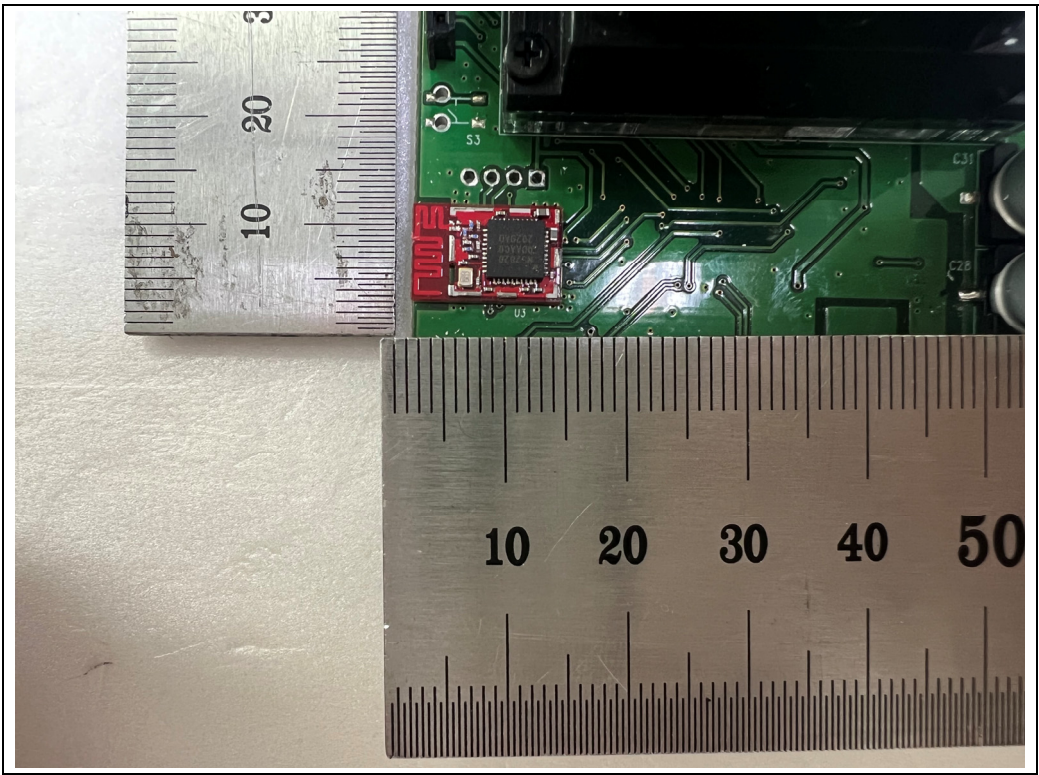
<Module&Antenna>
