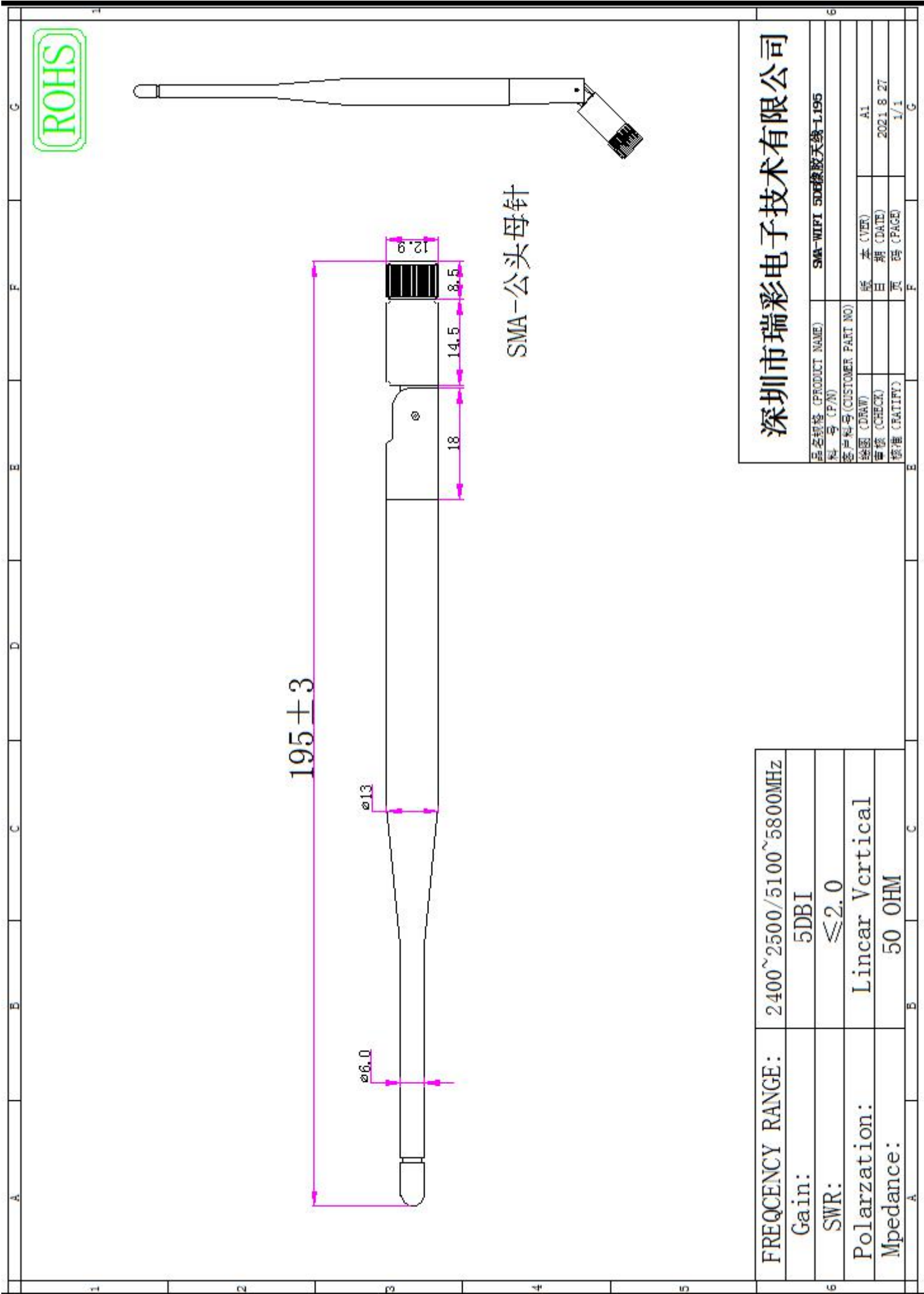
4.天线结构图:
