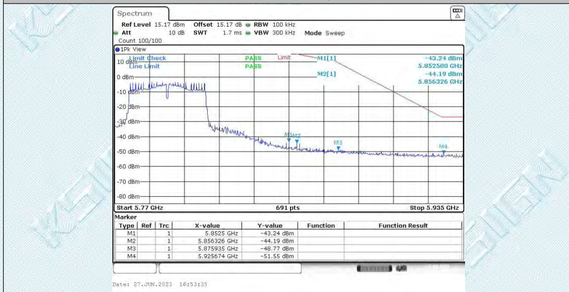
11AC80SISO_Ant1_Low_5775
