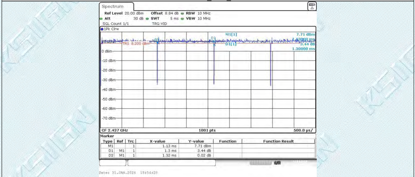
11N20SISO_Ant2_2437
