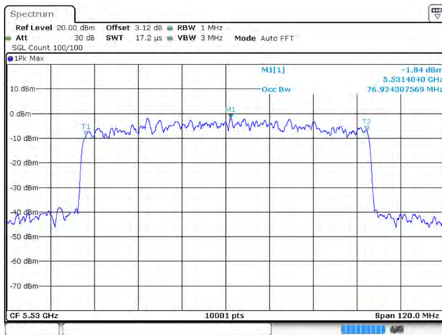
OBW ax80 5530MHz Ant2
