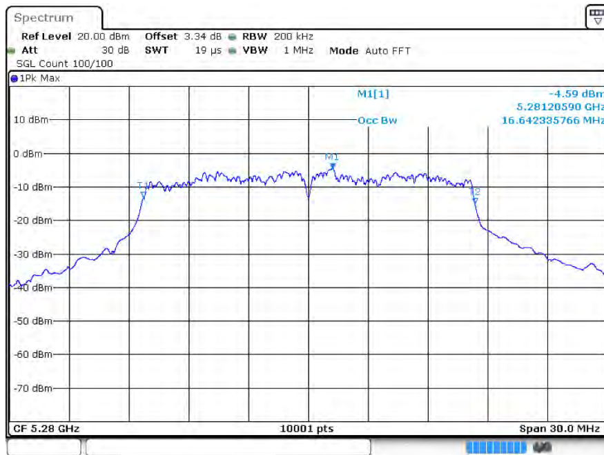
OBWa 5280MHz Ant2
