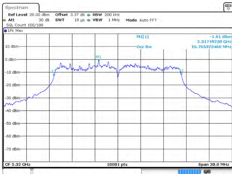
OBW a 5320MHz Ant2
