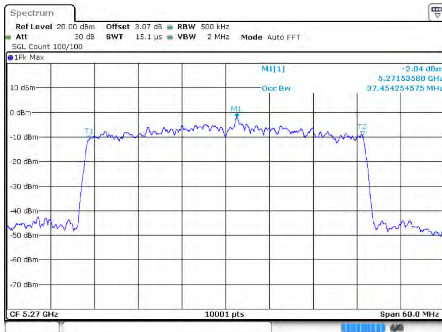
OBW ax40 5270MHz Ant1
