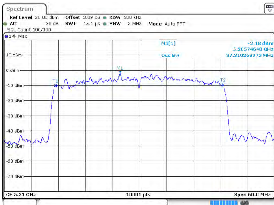
OBW ax40 5310MHz Ant1
