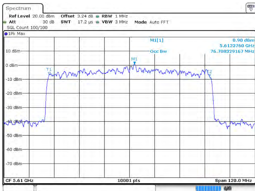
OBWax80 5610MHz Ant2
