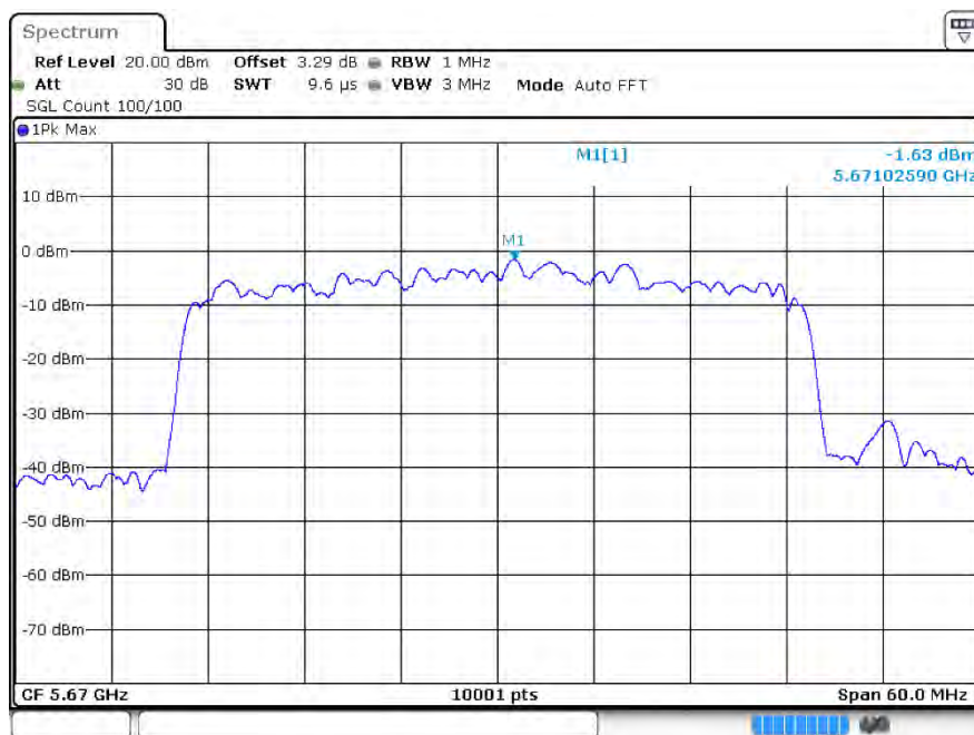
PSD ax40 5670MHz Ant1
