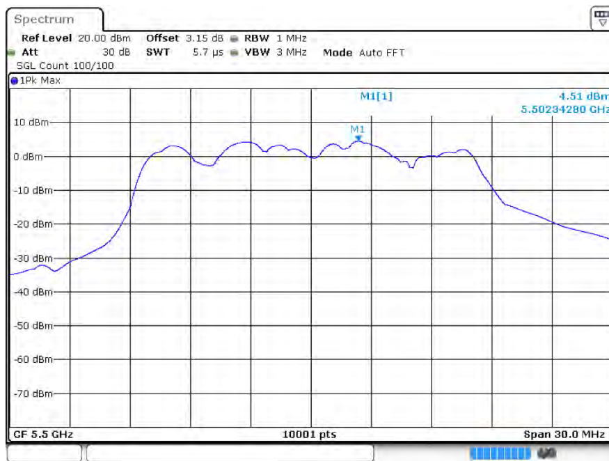
PSD ax20 5500MHz Ant1
