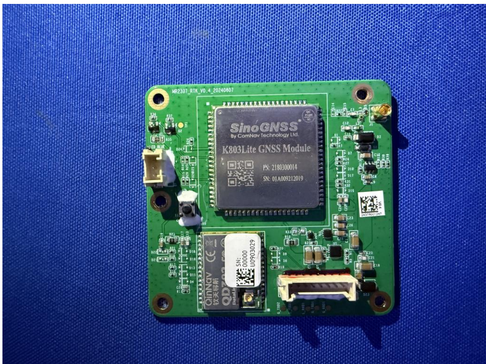
(36) EUT Photo
