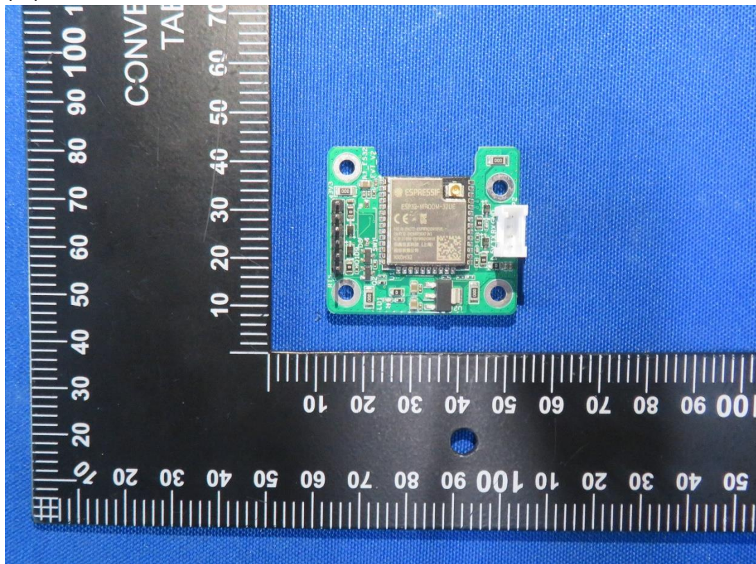
(14) EUT Photo
