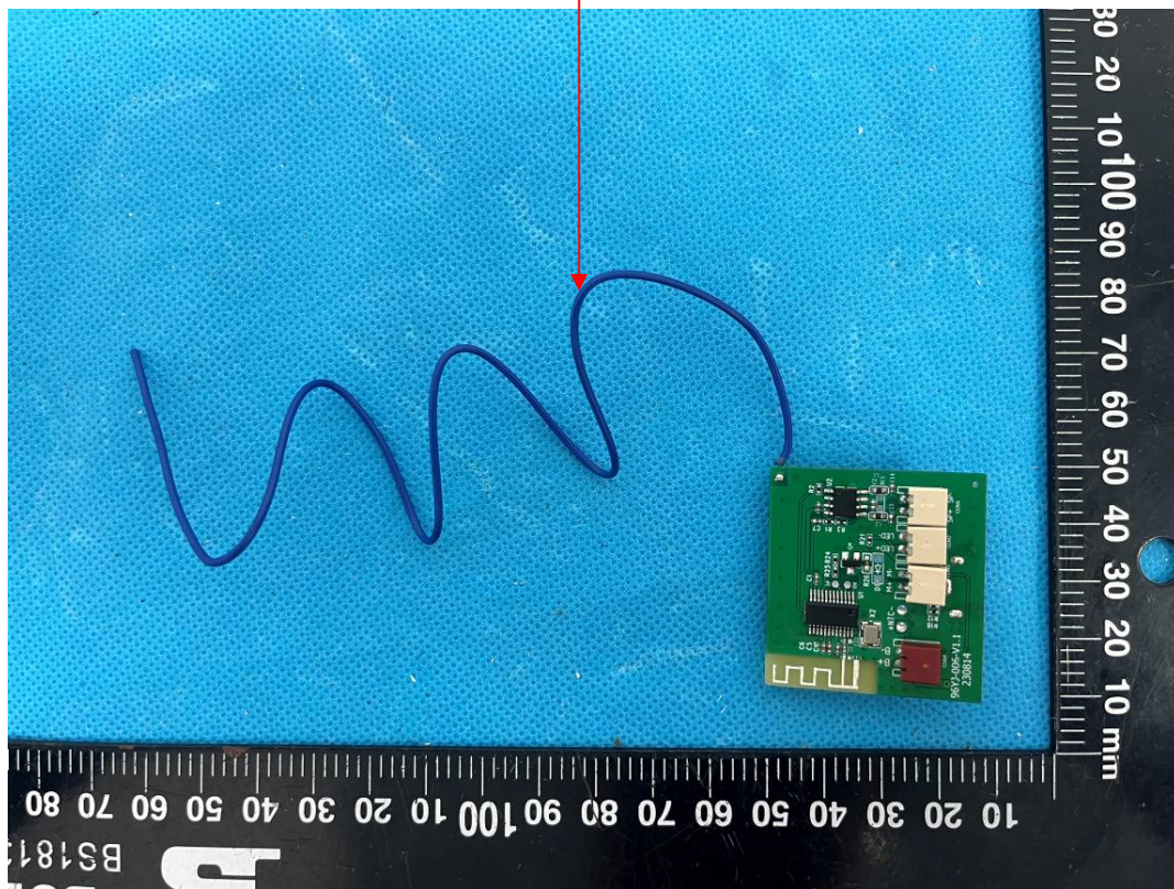
FM ANT
