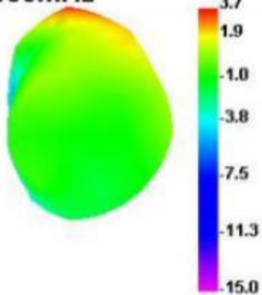
2450.000MHz
