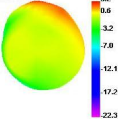
2400.000MHz
