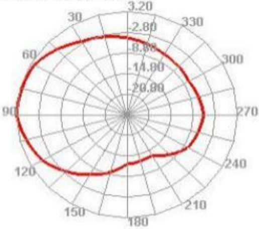
2400.000MHz H
