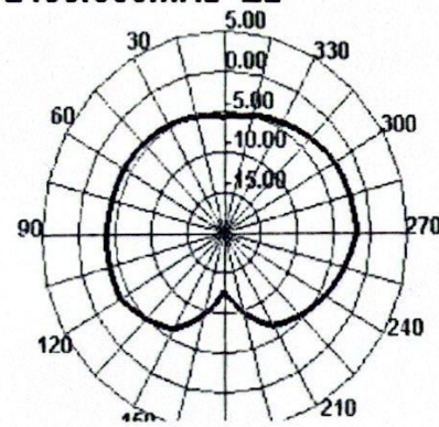
2450.000MHz E2
