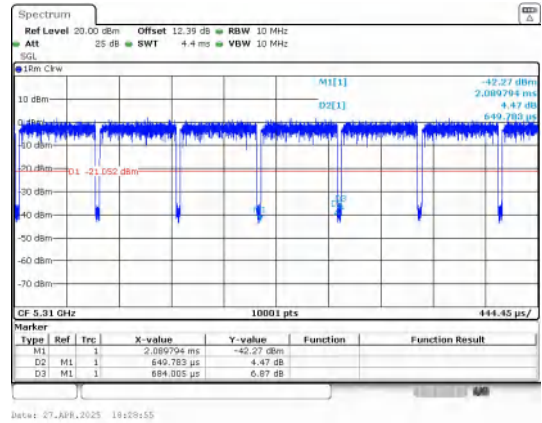
IEEE 802.11n_40MHz_Channel 62
