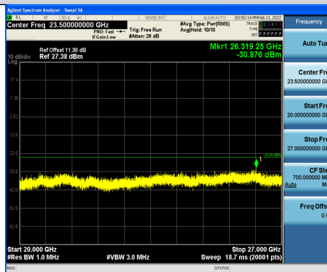
Band7-10MHz-QPSK-21100-1RB#0-Range3:20000~27000MHz
