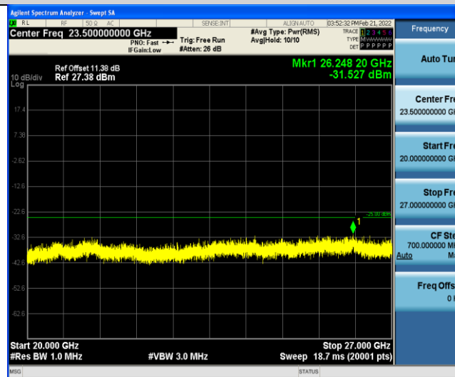
Band7-10MHz-QPSK-21400-1RB#0-Range3:20000~27000MHz
