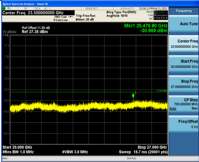
Band7-10MHz-QPSK-20800-1RB#0-Range5:20000~27000MHz
