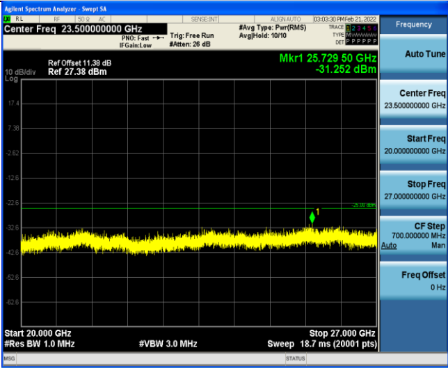
Band7-5MHz-QPSK-21100-1RB#0-Range5:20000~27000MHz
