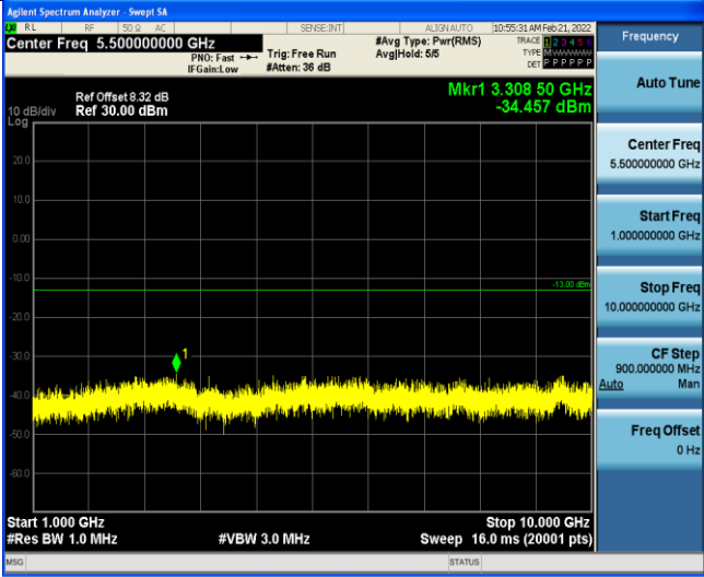
Band13-5MHz-QPSK-23230-1RB#0-Range2:1000~10000MHz
