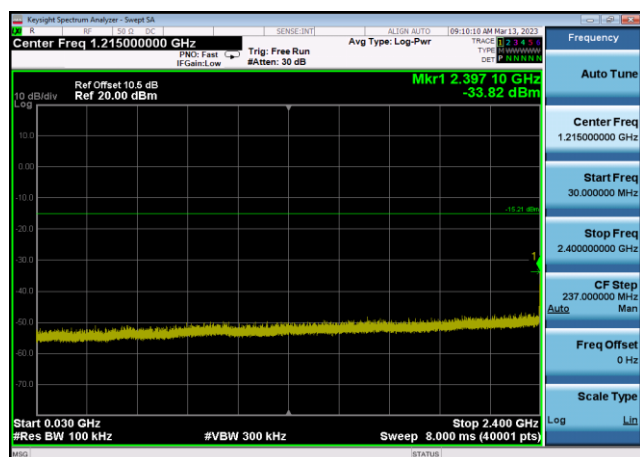
,Plot 3,30MHz~2400MHz-802.11b,2462MHz
