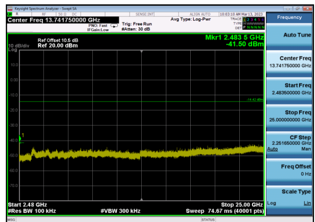
,Plot 4,2483.5MHz~25000MHz-802.11n(HT20),2462MHz,Ant0
