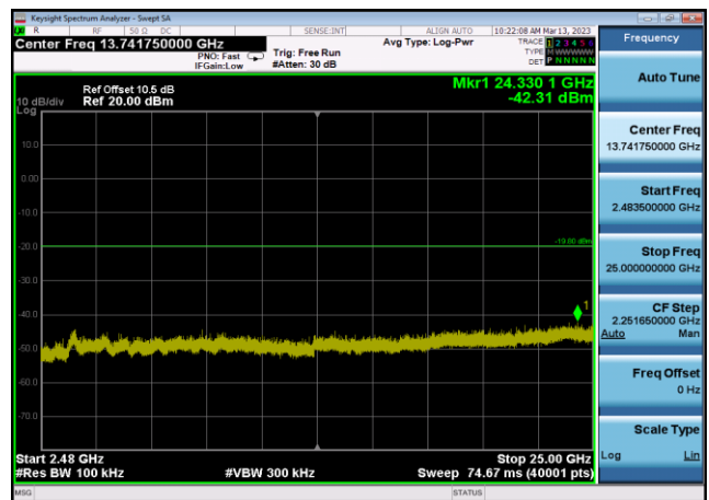
,Plot 4,2483.5MHz~25000MHz-802.11n(HT40),2452MHz,Ant0
