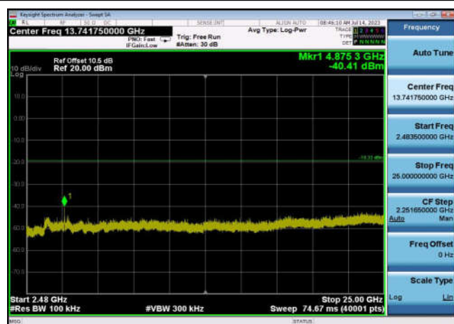
,Plot 4,2483.5MHz~25000MHz-802.11n(HT40),2437MHz,Ant0
