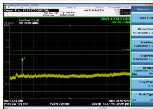
,Plot 4,2483.5MHz~25000MHz-802.11b
