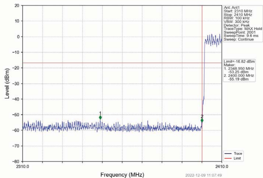
Pi/4DQPSK_2DH5_HOPP_Ant1_NTNV
