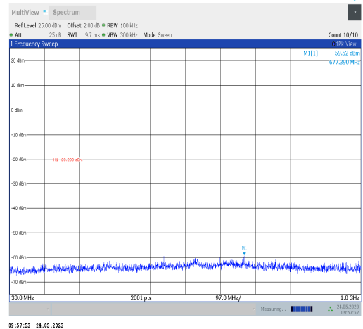
BLE_1M-Ant0-2480-30~1000
