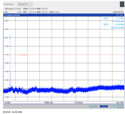
BLE_1M-Ant0-2440-1000~26500
