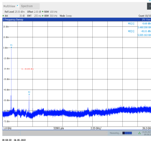
BLE_1M-Ant0-2480-1000~26500
