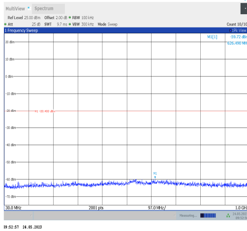
BLE_1M-Ant0-2440-30~1000
