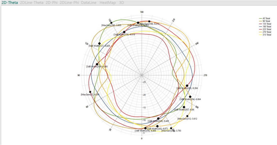
天线 2440MHz 2D-Theta Pattern
