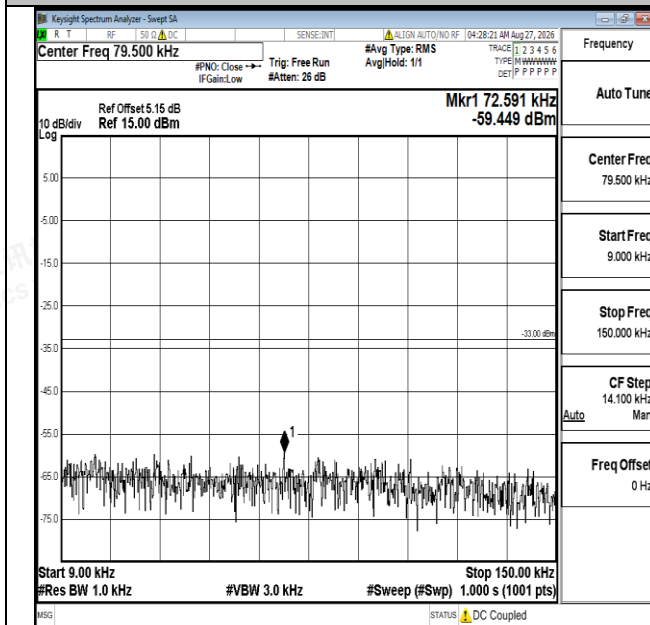
Band5-3MHz-QPSK-20635-1RB#0-0.009~0.15-PASS
