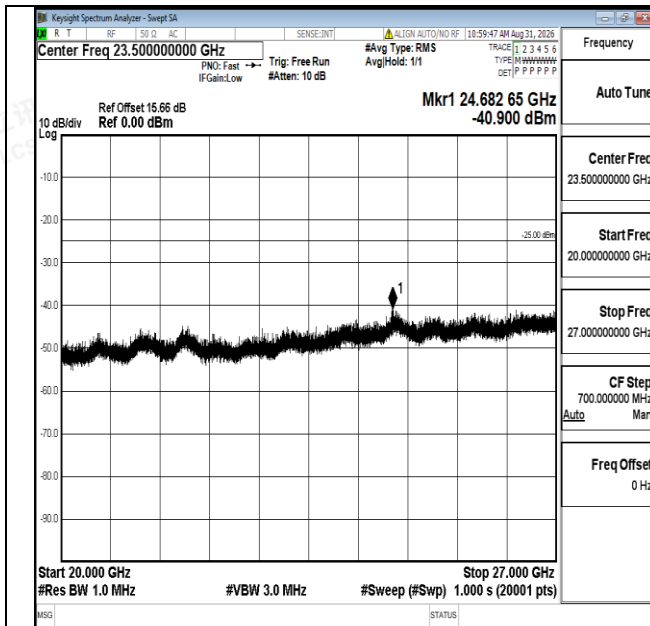
Band7-15MHz-QPSK-20825-1RB#0-20000~27000-PASS
