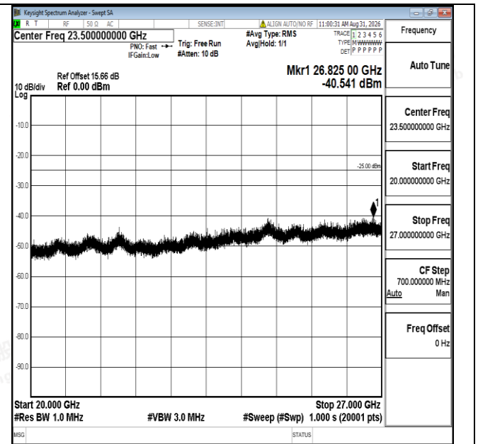
Band7-15MHz-16QAM-20825-1RB#0-20000~27000-PASS
