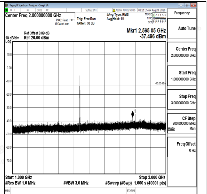
Band25-10MHz-QPSK-26365-1RB#0-1000~3000-PASS
