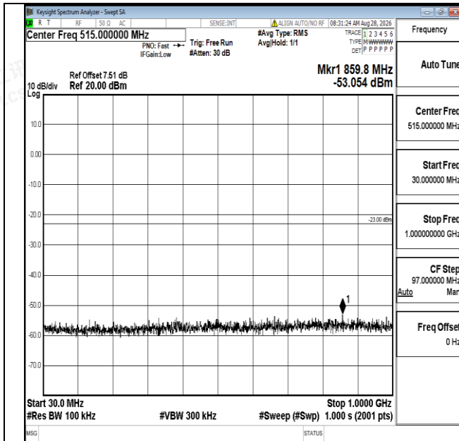
Band25-10MHz-QPSK-26365-1RB#0-30~1000-PASS
