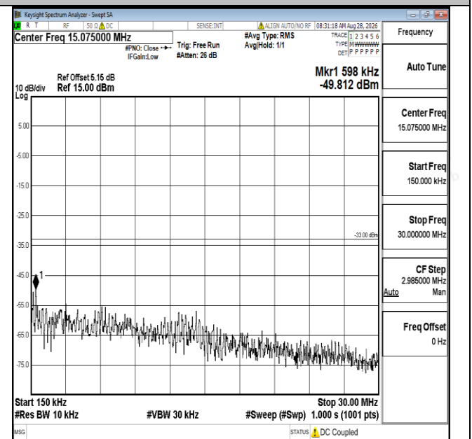
Band25-10MHz-QPSK-26365-1RB#0-0.15~30-PASS
