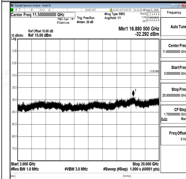
Band25-15MHz-QPSK-26115-1RB#0-3000~20000-PASS
