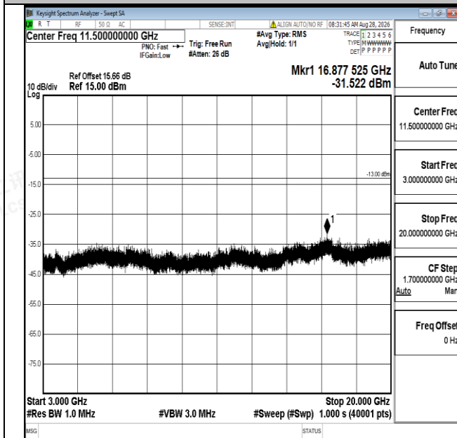
Band25-10MHz-QPSK-26365-1RB#0-3000~20000-PASS
