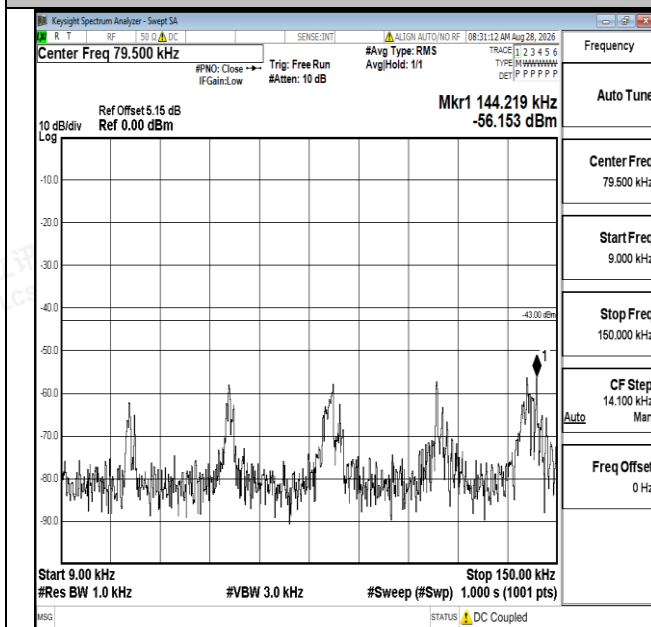
Band25-10MHz-QPSK-26365-1RB#0-0.009~0.15-PASS
