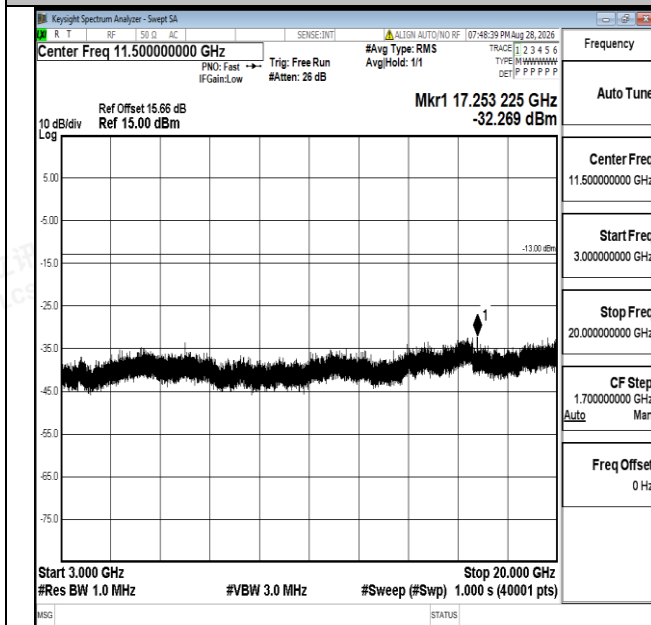
Band25-20MHz-QPSK-26365-1RB#0-3000~20000-PASS
