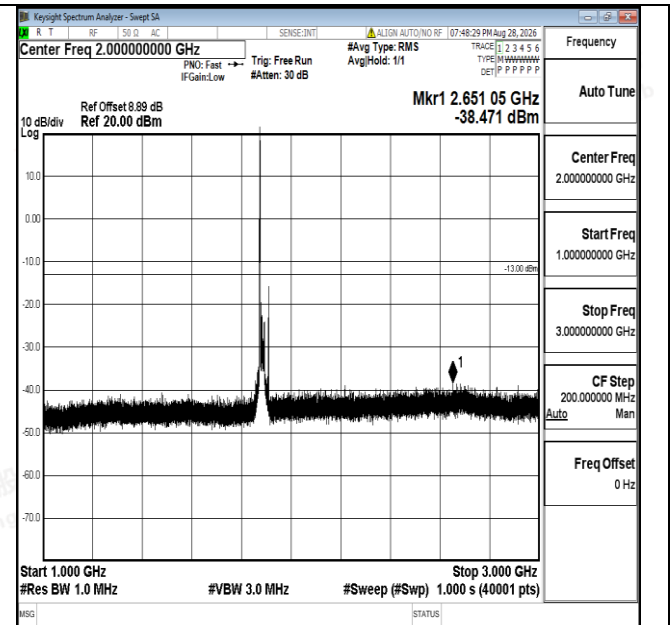
Band25-20MHz-QPSK-26365-1RB#0-1000~3000-PASS
