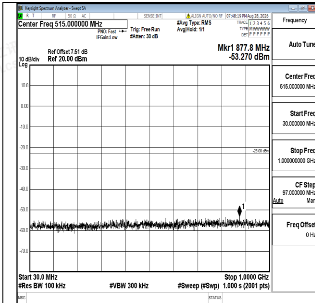
Band25-20MHz-QPSK-26365-1RB#0-30~1000-PASS
