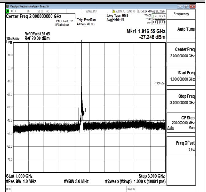
Band25-20MHz-QPSK-26590-1RB#0-1000~3000-PASS
