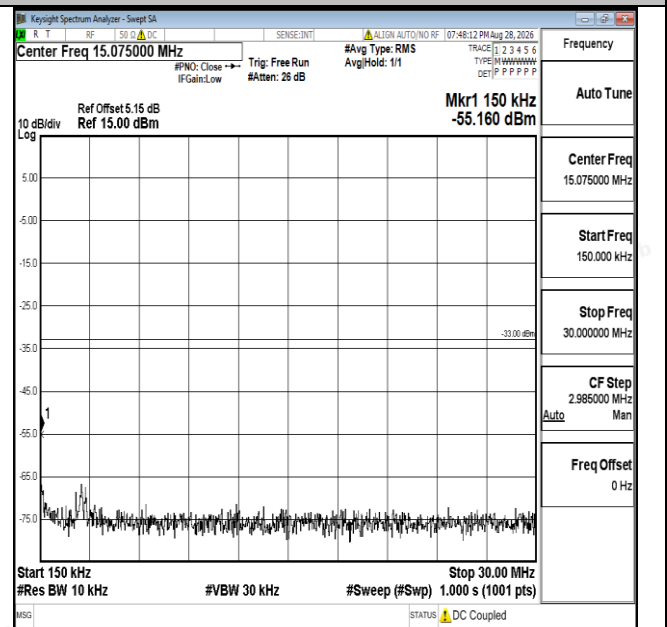
Band25-20MHz-QPSK-26365-1RB#0-0.15-30-PASS
