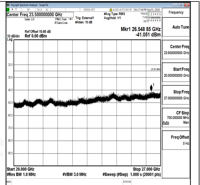
Band38-15MHz-16QAM-37825-1RB#0-20000~27000-PASS
