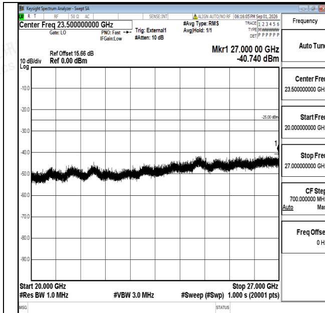
Band38-15MHz-QPSK-37825-1RB#0-20000~27000-PASS
