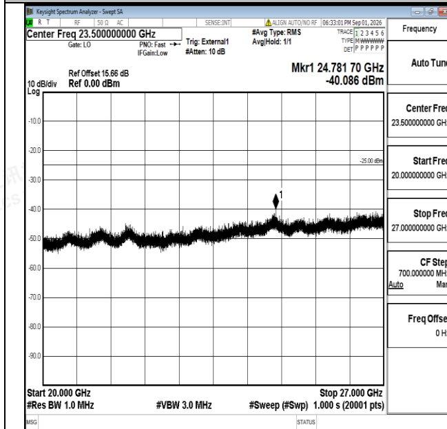
Band38-20MHz-QPSK-38150-1RB#0-20000~27000-PASS
