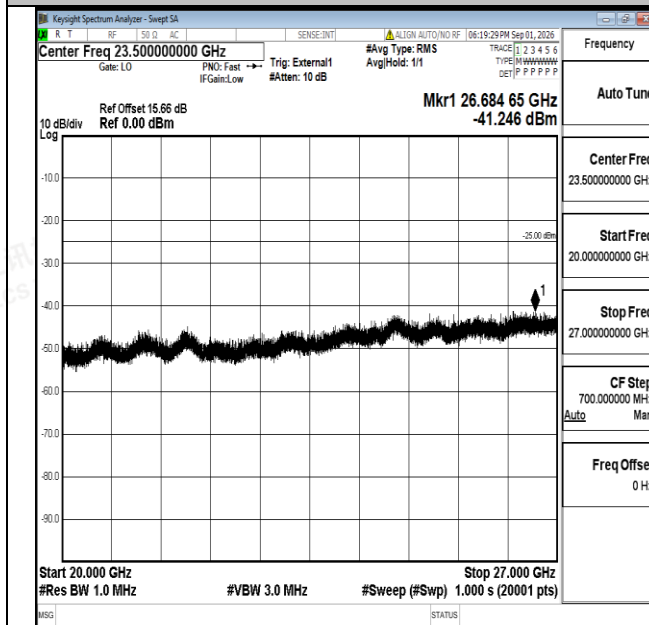
Band38-15MHz-QPSK-38000-1RB#0-20000~27000-PASS
