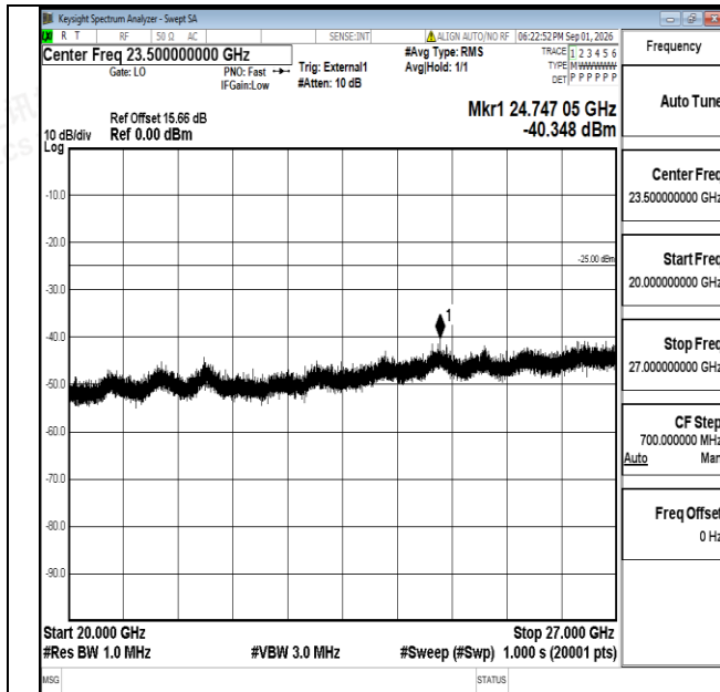
Band38-15MHz-QPSK-38175-1RB#0-20000~27000-PASS
