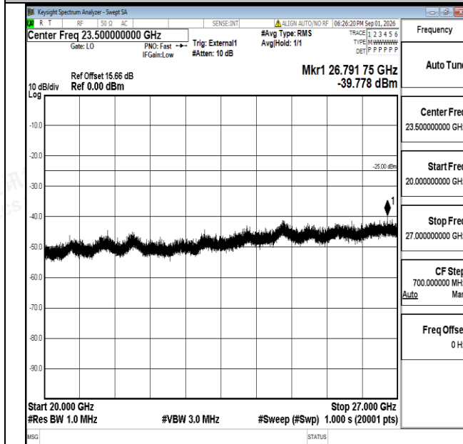
Band38-20MHz-QPSK-37850-1RB#0-20000~27000-PASS
