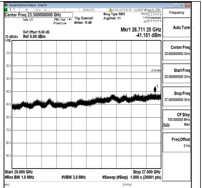
Band41-5MHz-16QAM-41565-1RB#0-20000~27000-PASS
