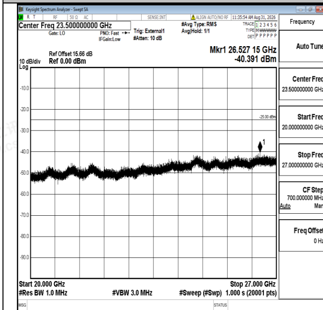
Band41-10MHz-QPSK-41540-1RB#0-20000~27000-PASS
