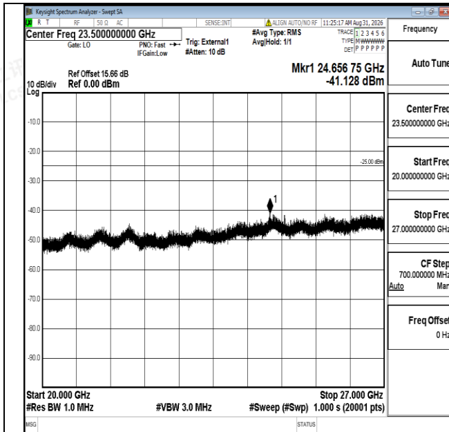
Band41-5MHz-QPSK-41565-1RB#0-20000~27000-PASS
