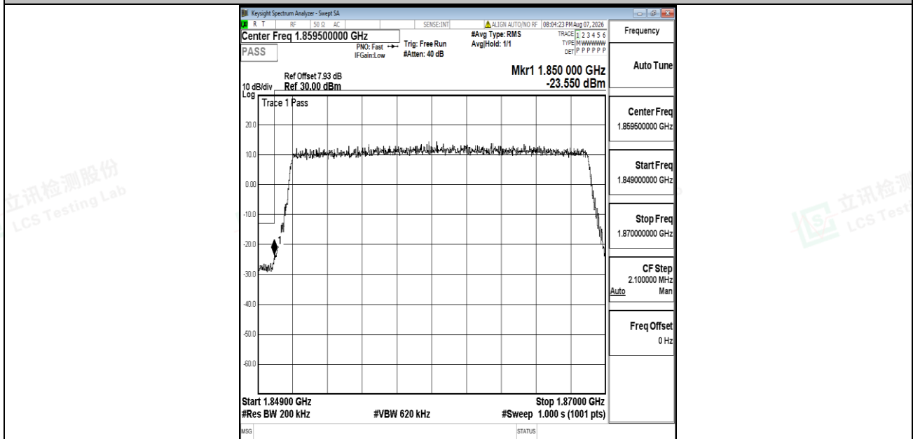
Band2-20MHz-16QAM-18700-100RB#0-PASS
