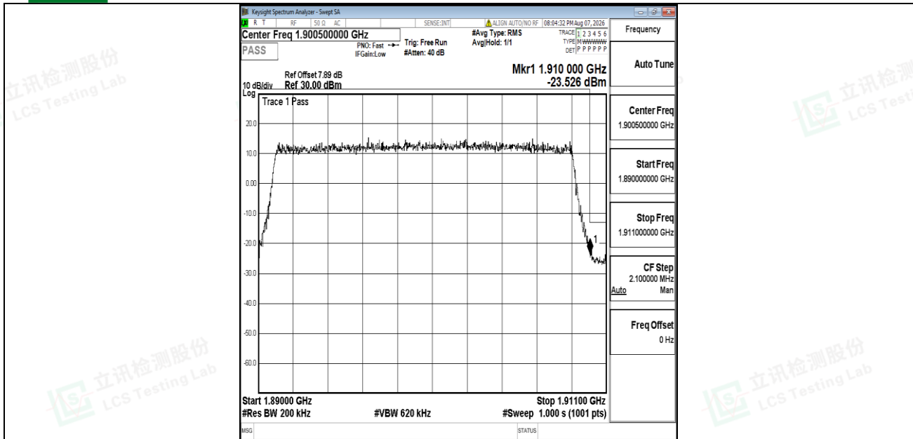
Band2-20MHz-QPSK-19100-100RB#0-PASS
