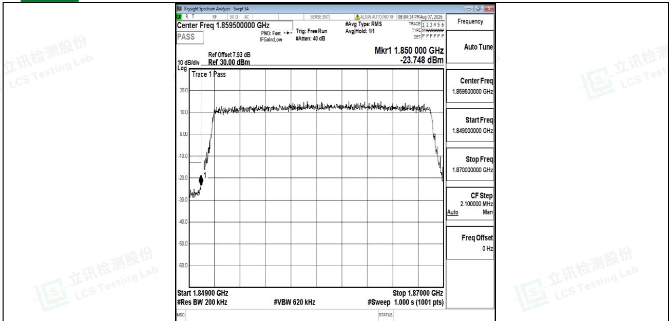
Band2-20MHz-QPSK-18700-100RB#0-PASS
