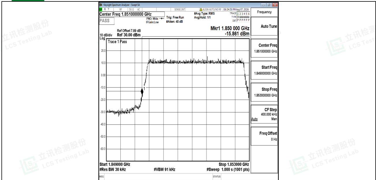
Band2-3MHz-QPSK-18615-15RB#0-PASS
