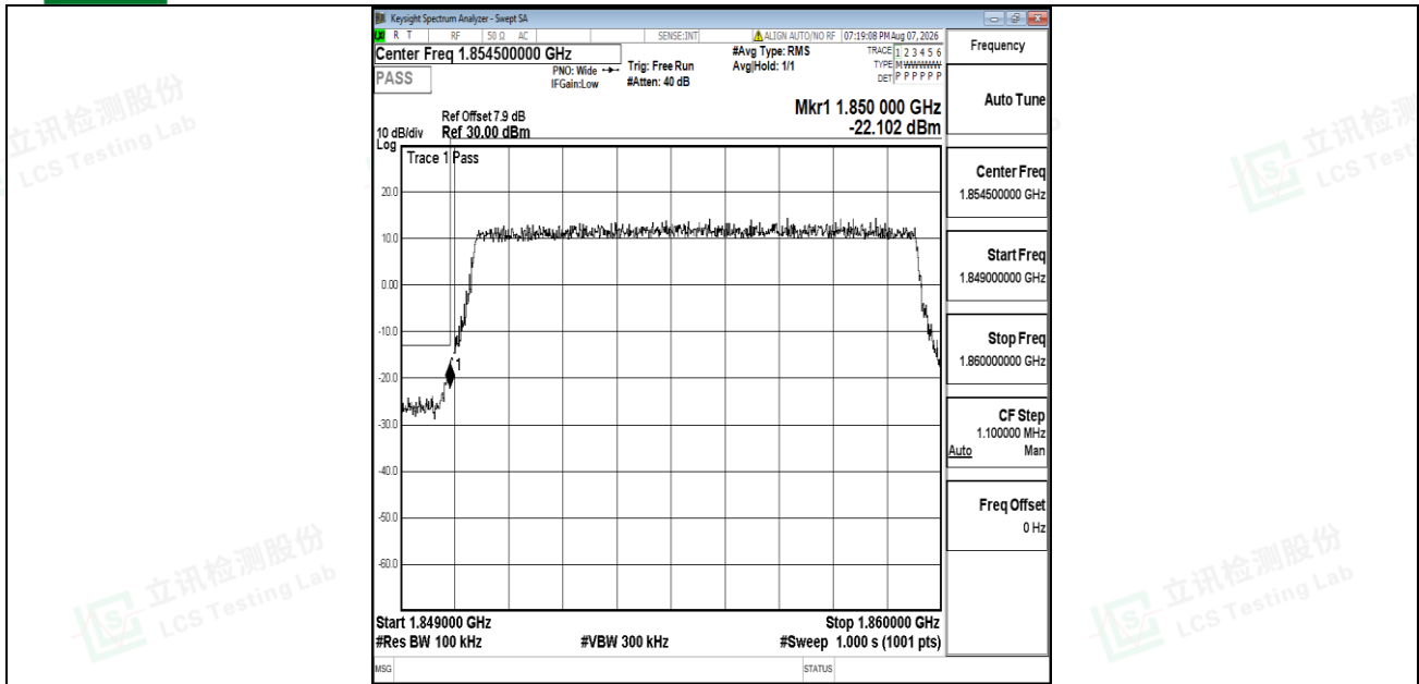
Band2-10MHz-QPSK-18650-50RB#0-PASS
