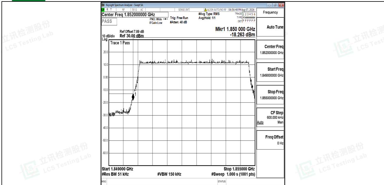
Band2-5MHz-QPSK-18625-25RB#0-PASS
