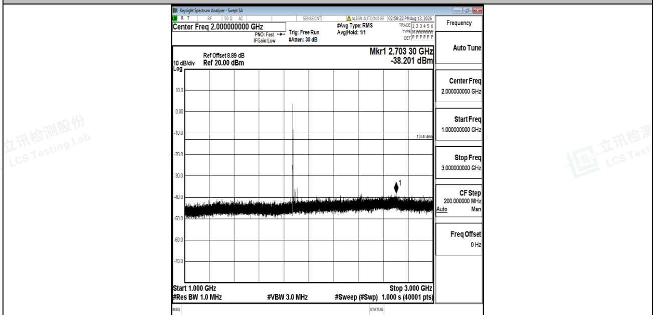
Band2-20MHz-QPSK-18900-1RB#0-1000~3000-PASS
