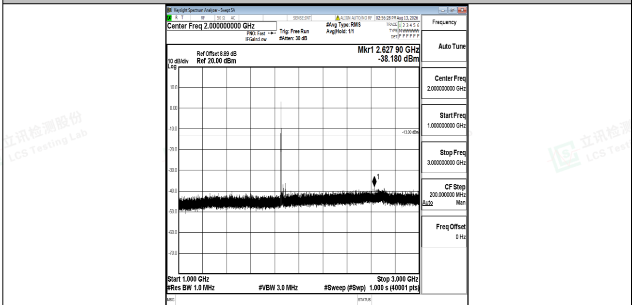
Band2-20MHz-QPSK-18700-1RB#0-1000~3000-PASS
